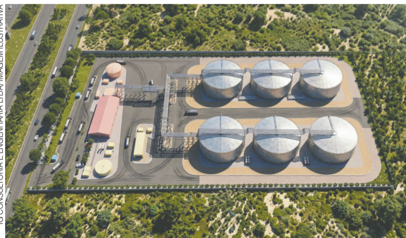
Usina de Hidrogênio Verde do projeto Morro Pintado, em Areia Branca, no RN
